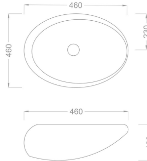
TEKNİK ÇİZİM
