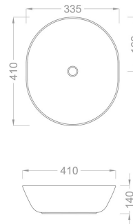
TEKNİK ÇİZİM
