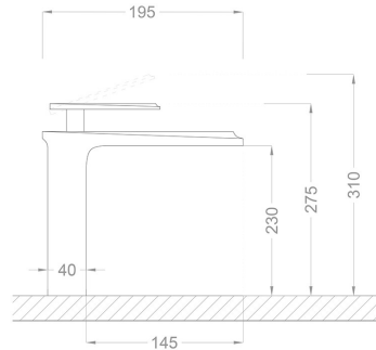
TEKNİK ÇİZİM
