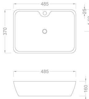
TEKNİK ÇİZİM
