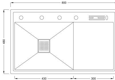
TEKNİK ÇİZİM
