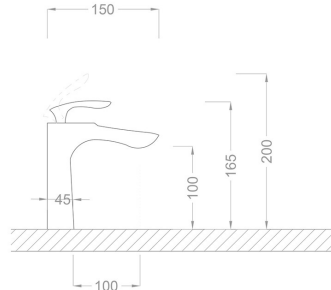
TEKNİK ÇİZİM
