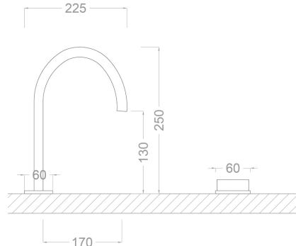
TEKNİK ÇİZİM
