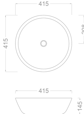
TEKNİK ÇİZİM
