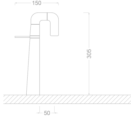
TEKNİK ÇİZİM
