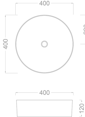
TEKNİK ÇİZİM
