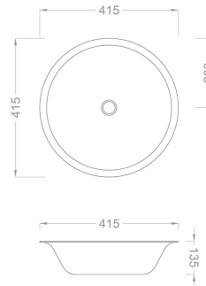
TEKNİK ÇİZİM
