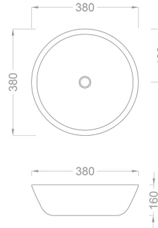
TEKNİK ÇİZİM
