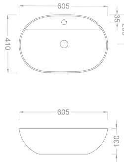
TEKNİK ÇİZİM
