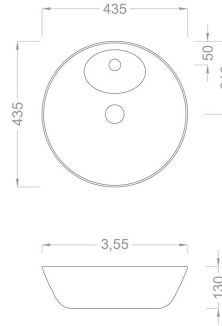
TEKNİK ÇİZİM
