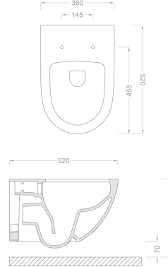
TEKNİK ÇİZİM
