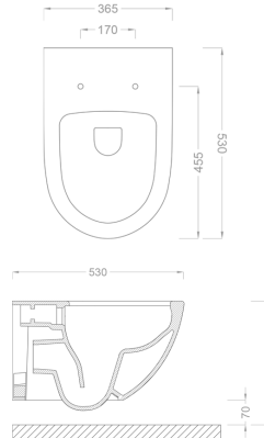
TEKNİK ÇİZİM
