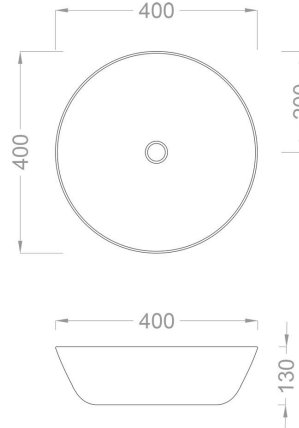
TEKNİK ÇİZİM
