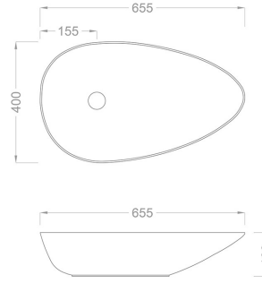
TEKNİK ÇİZİM
