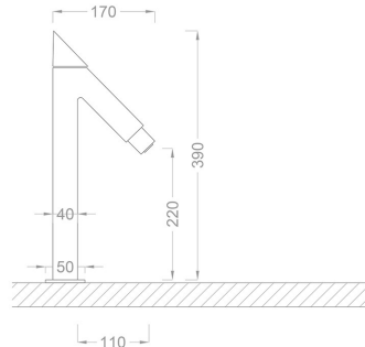
TEKNİK ÇİZİM
