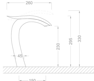
TEKNİK ÇİZİM
