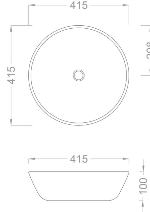
TEKNİK ÇİZİM
