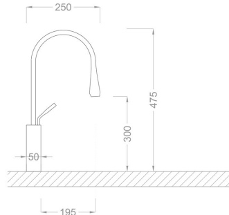
TEKNİK ÇİZİM
