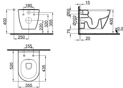
TEKNİK ÇİZİM
