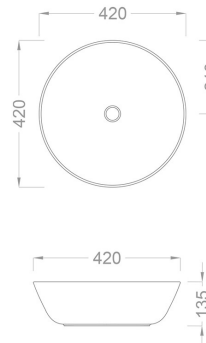
TEKNİK ÇİZİM
