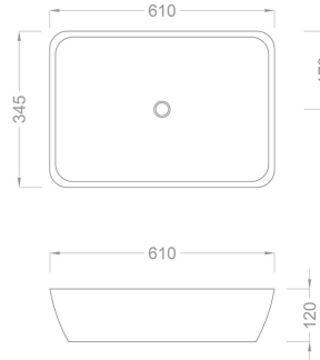
TEKNİK ÇİZİM
