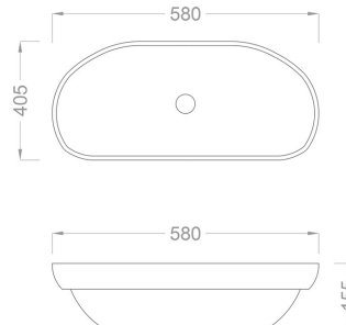
TEKNİK ÇİZİM
