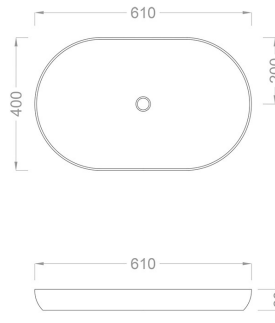
TEKNİK ÇİZİM
