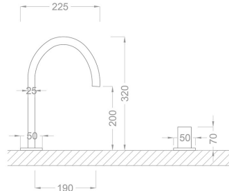
TEKNİK ÇİZİM
