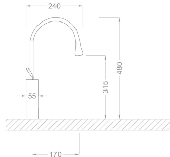
TEKNİK ÇİZİM
