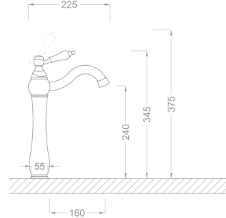
TEKNİK ÇİZİM
